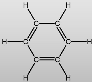
Benzol
